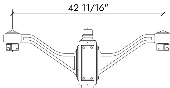
Richmond Twin Pendant
