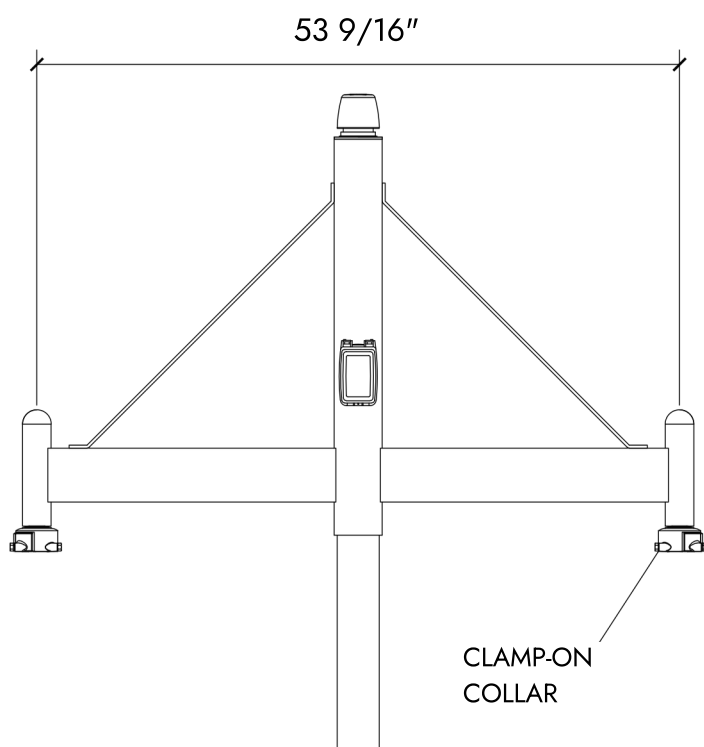
Contempo Twin Pendant
