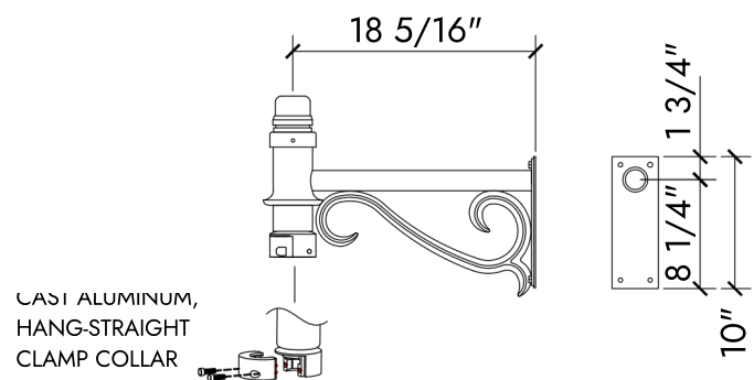
Colonial Pendant Bracket
